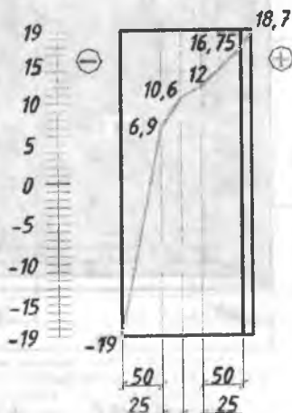
Рис. 7. Розподіл температур в перерізі еталонного зразка /
