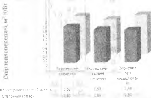
Рис. 8. Порівняння значень опору теплопередачі в експериментальних зразках /
