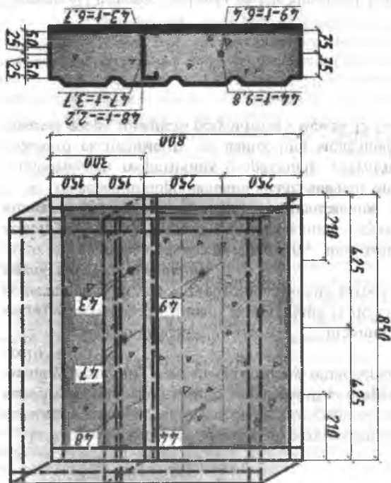
Рис. 4. Схема розміщення термопар для зразка з теплопровідним включенням (43-48 – № термопар) / The layout of thermocouples for specimen with thermal conductivity inclusion (43-48 – No thermocouples)
