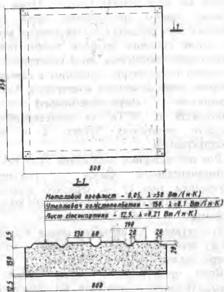
Рис. 2. Конструктивна схема термічно однорідної стінової панелі /
