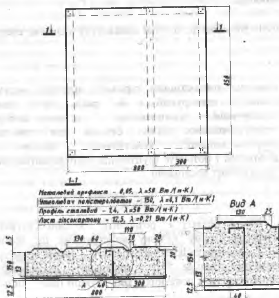
Рис. 1. Конструктивна схема стінової панелі з теплопровідним включенням /
