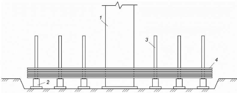
Рис. 2. Зведення будівлі методом підйому перекриттів:
