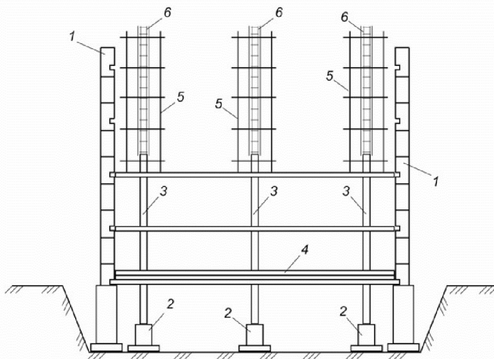
Рис. 4. Влаштування вбудованого каркасу методом підйому перекриттів (стадія бетонування колон другого ярусу):
