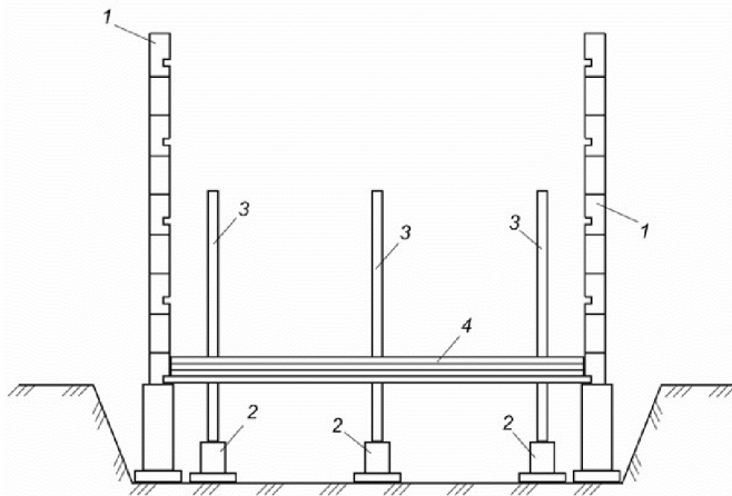
Рис. 3. Влаштування вбудованого каркасу методом підйому перекриттів (стадія бетонування плит перекриття):
