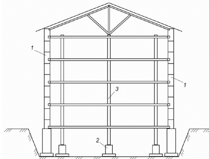
Рис. 1. Реконструкція будівлі за допомогою вбудованої системи:
