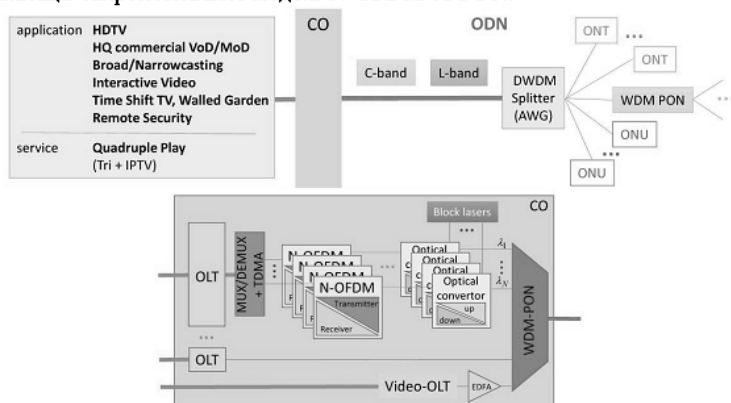
Рис. 1. Варіант гібридної N-OFDM-X-PON
