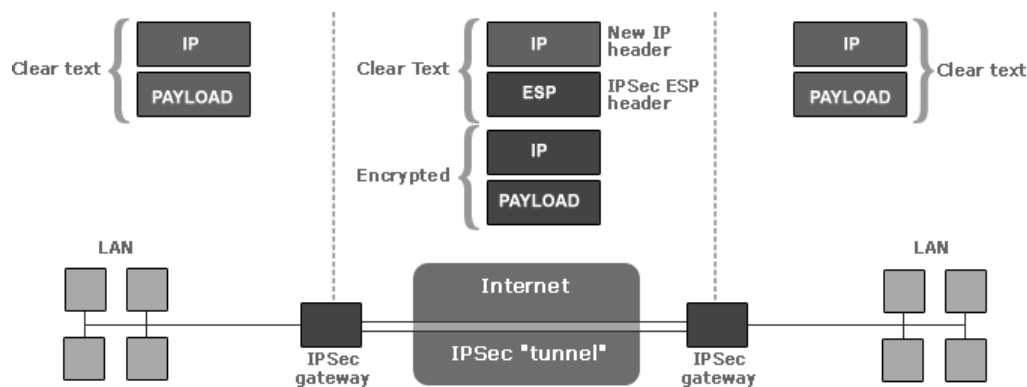
Рис. 1. Візуальне представлення реалізації IPsec для забезпечення безпечного зв'язку
