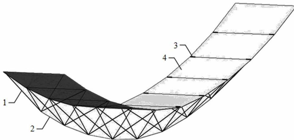
Рисунок 2 – Структурно-вантові сталезалізобетонні конструкції покриттів: а) балкова структурно-вантова конструкція; б) аркова структурно-вантова конструкція; в) структурно-вантова висяча система;
